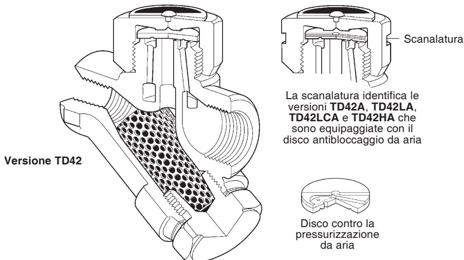
Fig. 1 Scaricatore termodinamico TD42 e relative versioni
